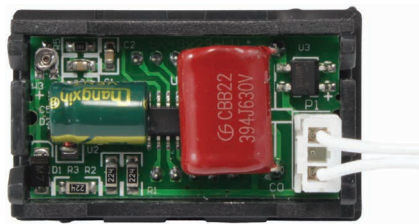
Рис. 2 – Вид сзади с подключенными входным сигналом и питанием
