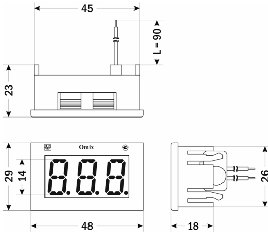
Рис. 3 – Размеры прибора
